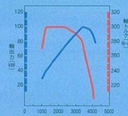
3.0L TDIディーゼルエンジン 1KD-FTV性能曲線図 総排気量: 2.982L 最高出力(ネット): 100kW (136PS) / 3,400r.p.m. 最大トルク(ネット): 300N·m (30.6kgf·m) / 1,200~2,400r.p.m.
